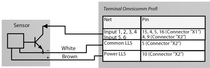
Рисунок 14. Схема подключения датчика с выходом N-P-N типа «открытый коллектор»
