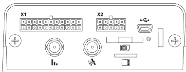
Рисунок 1. Общий вид терминала Omnicomm Profi
