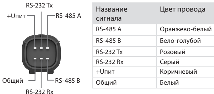
Рисунок 3. Разъем датчика Omnicomm LLS 4
