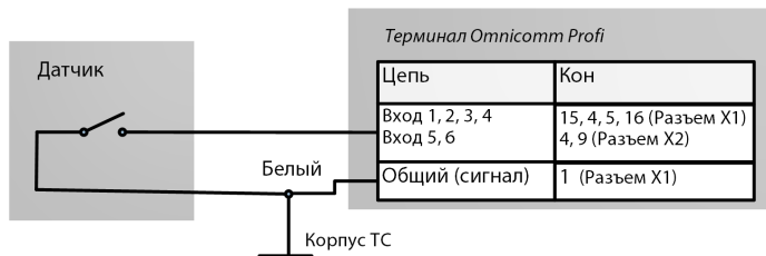
Рисунок 15. Схема подключения контактного датчика
