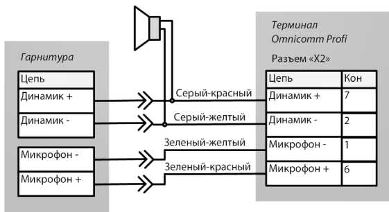
Рисунок 9. Схема подключения комплекта голосовой связи
