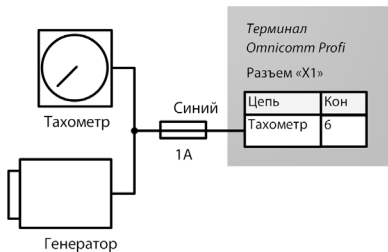
Рисунок 7. Схема подключения к тахометру
