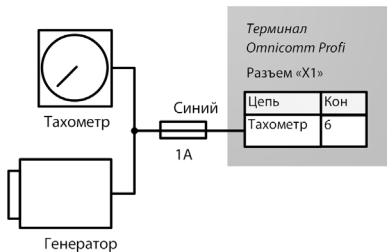
Рисунок 7. Схема подключения к тахометру
