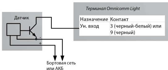
Рисунок 10. Схема подключения датчика с выходом N-P-N типа «открытый коллектор»
