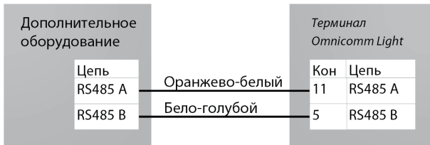
Рисунок 6. Схема подключения оборудования по интерфейсу RS-485
