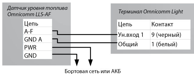
Рисунок 13. Схема подключения датчика уровня топлива Omnicomm LLS-AF
