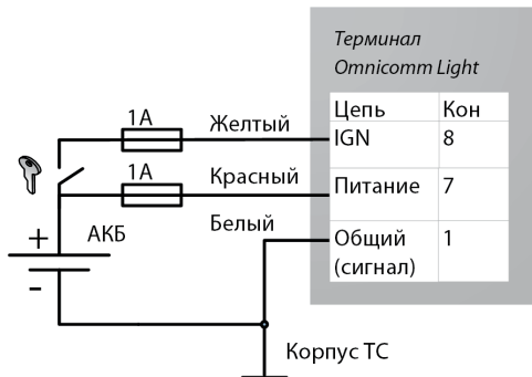
Рисунок 3. Схема подключения на ТС без прерывателя «массы»
