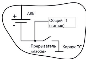
Рисунок 5. Схема подключения на ТС до прерывателя «массы»
