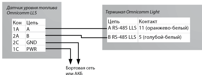
Рисунок 12. Схема подключения датчика уровня топлива Omnicomm LLS
